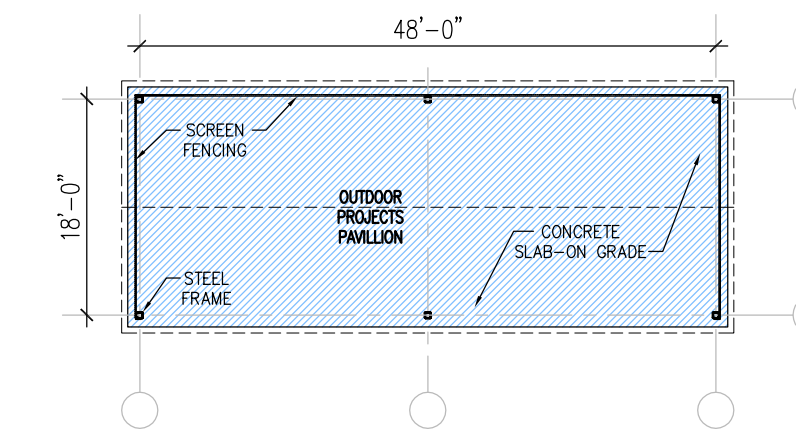
Pavillion Plan SCALE: 1/8" = 1'-0"
